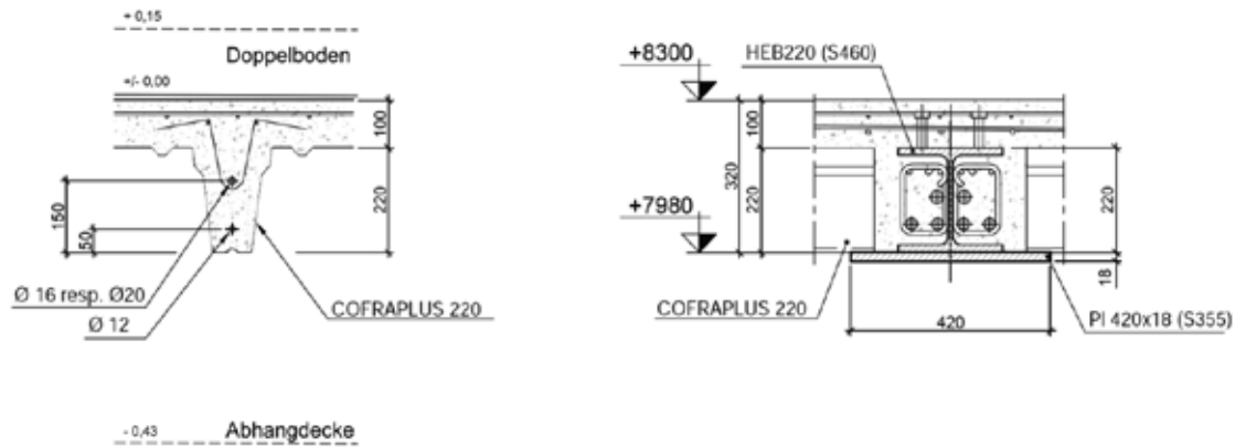
„Bild 10. Querschnitt des Verbunddeckensystems und der Slim-Floor-Träger inklusive Brandschutzbewehrung (Quelle: Schroeder & Associés)
